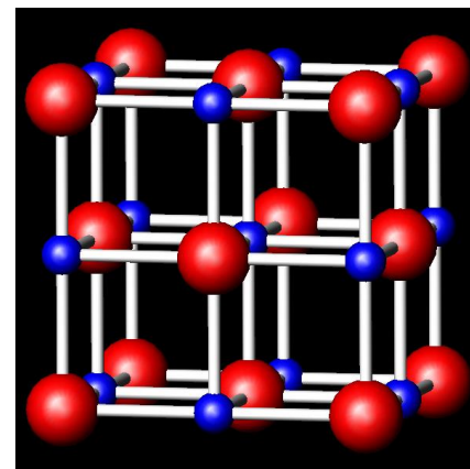
NiO
