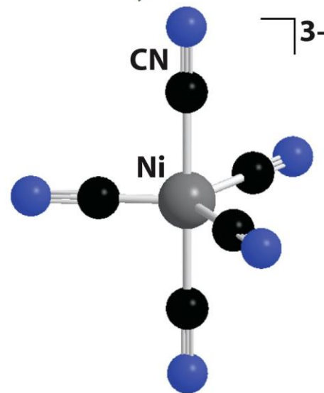
тригональная бипирамида
