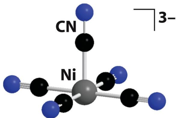
квадратная пирамида
