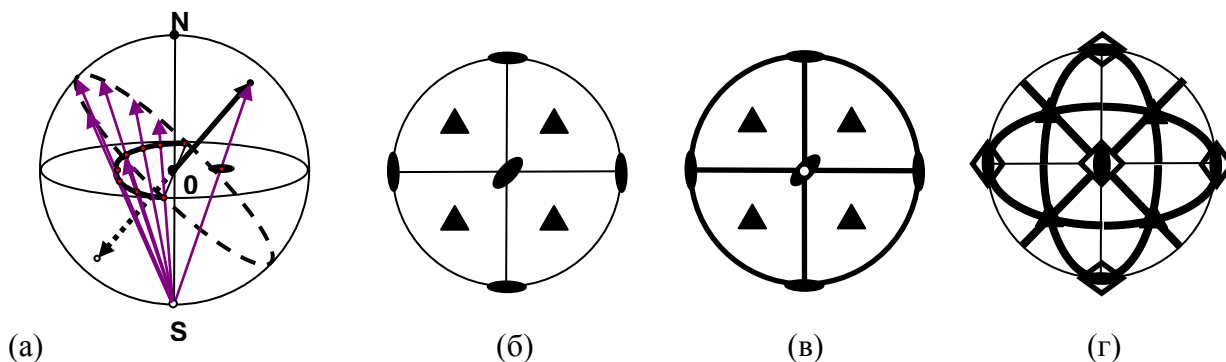
Рис. 1.10. (а) Изображение наклонных элементов симметрии на стереографической проекции и графики групп семейства тетраэдра: 23 (б) m\bar{3} (в) и 4\bar{3}m (г)
