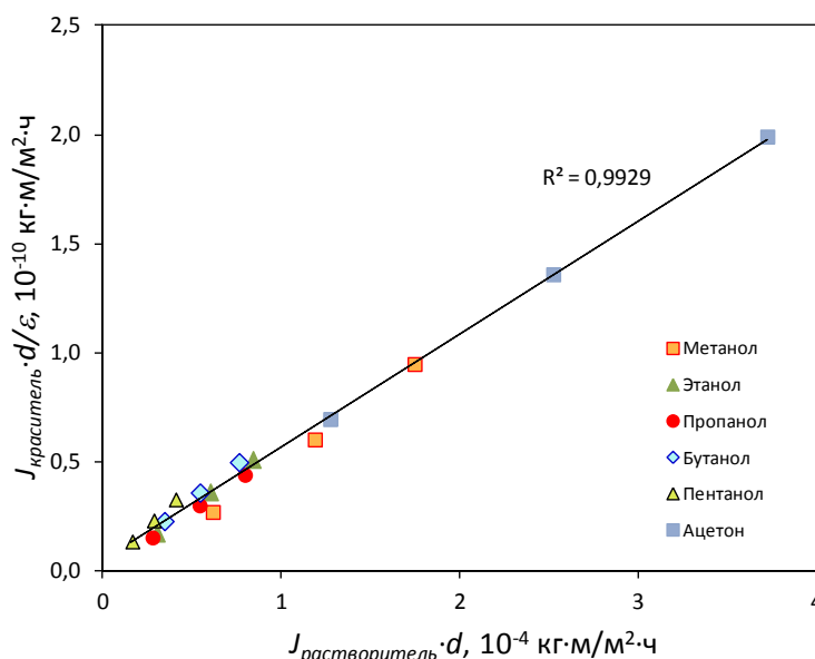
Рисунок 6. Соотношение потока растворителя и маркера Solvent Blue 35 в мембране ПТМСП при давлениях 10, 20 и 30 атм. с учетом полярности растворителя (диэлектрическая постоянная \varepsilon ).
