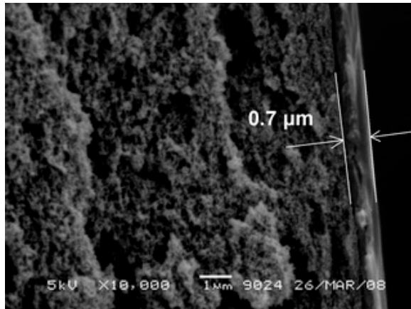
г – ПТМСП-11
