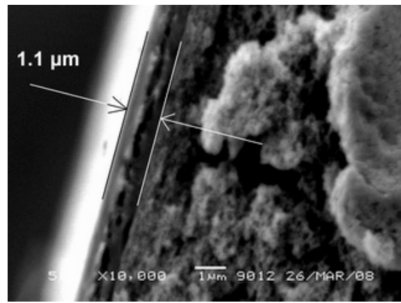
б – ПТМСП-9
