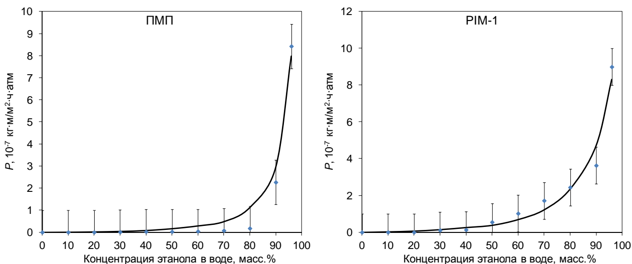
Рисунок 5. Зависимость коэффициента проницаемости жидкости P от состава исходной смеси вода-этанол для сплошных мембран из ПМП и PIM-1 ( \Delta p=20 атм).
