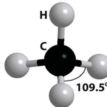
метан CH 4
