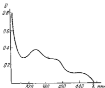
Рис 11 Светопоглощение 4-метилпио ксидата никеля в толуоле
