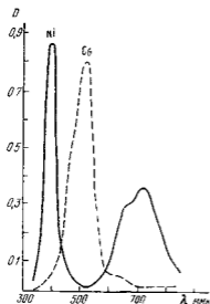
Рис 27 Светопоглощение перхлоратов никеля и кобальта
