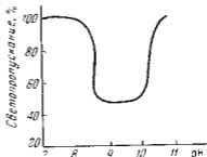
Рис 21 Образование меркаптопропионата никеля в зависимости от значения pH водного раствора
