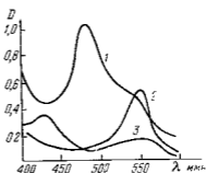
Рис. 7. Светопоглощение суспензий диоксида никеля.
