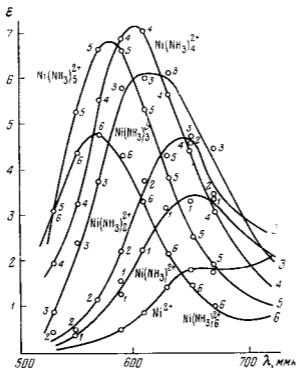
Рис 1 Светопоглощение аммиаков никеля в 2 N растворе нитрата аммония при 23° С Цифры соответствуют числу молекул аммиака в комплексах
