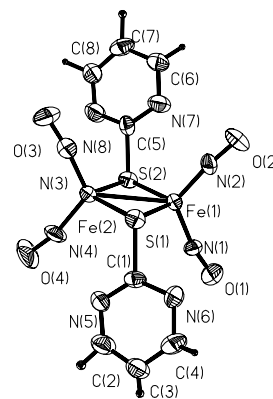
Рис. 4. Кристаллическое строение [\text{Fe}_2(\text{SC}_4\text{H}_3\text{N}_2)_2(\text{NO})_4]
