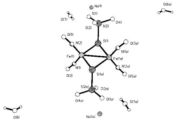
Рис. 2. Кристаллическое строение комплекса \text{Na}_2[\text{Fe}_2(\text{S}_2\text{O}_3)_2(\text{NO})_4] \cdot 4\text{H}_2\text{O}
